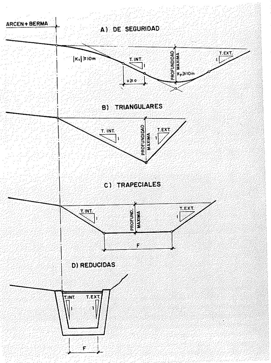
Fig. 3.10. CUNETAS
