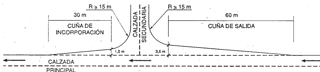
Figura 7.3 Cuñas de cambio de velocidad.
